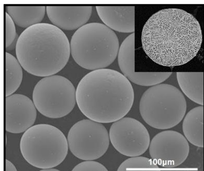
■ガスアトマイズ粉末の電子顕微鏡写真 およびミクロ組織
