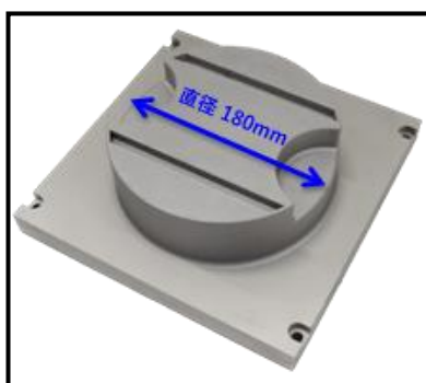
■開発品 金型向け金属粉末 S-MEC®シリーズ 「S-MEC®34D」（高熱伝導性工具鋼粉末） による大型造形例
