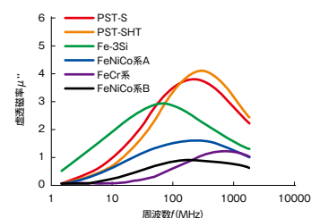
(b-2) 標準粒径タイプ虚透磁率 \mu''
