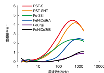
(b-1) 小粒径タイプ虚透磁率 \mu''
