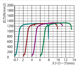
常温引張試験における Inconel718造形体の応力-ひずみ曲線測定例
