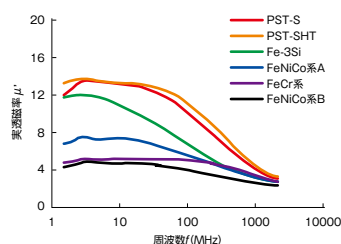
(a-2) 標準粒径タイプ実透磁率 \mu'
