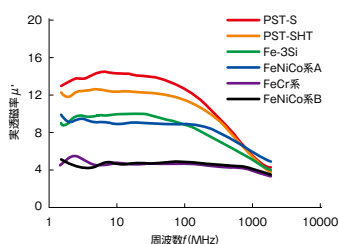
(a-1) 小粒径タイプ実透磁率 \mu'
