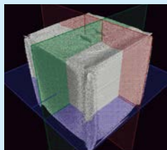
Co基合金造形体の 内部欠陥解析例
