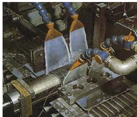
突っ切り切断機 Tube cutting machine
