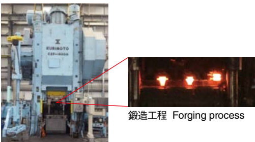
ホット鍛造プレス 1600t Hot vertical press 1600t
